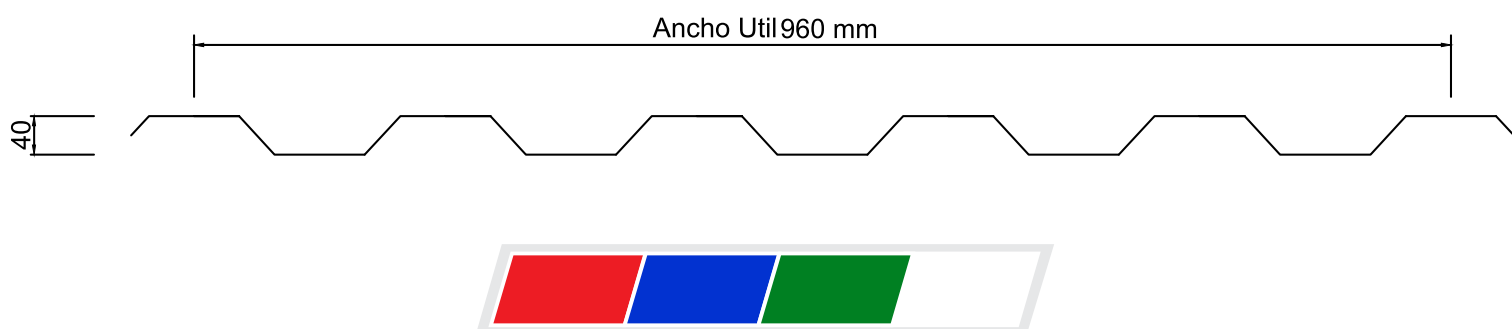
Perfil TTR-6B
